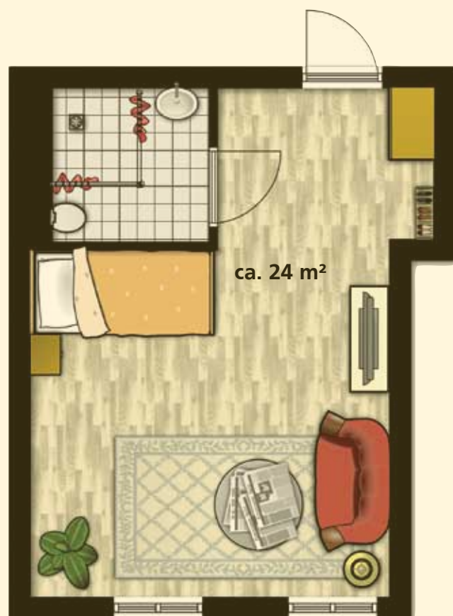
Variante Einzelzimmer
